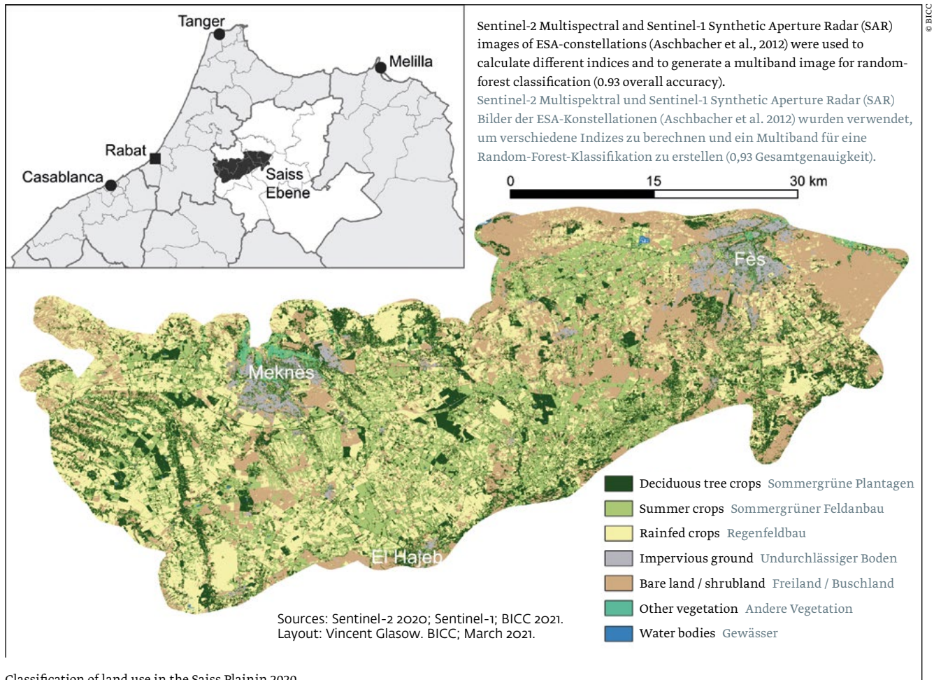
Classification of land use in the Saiss Plain in 2020 Landnutzungsklassifikation der in der Saiss-Ebene 2020
